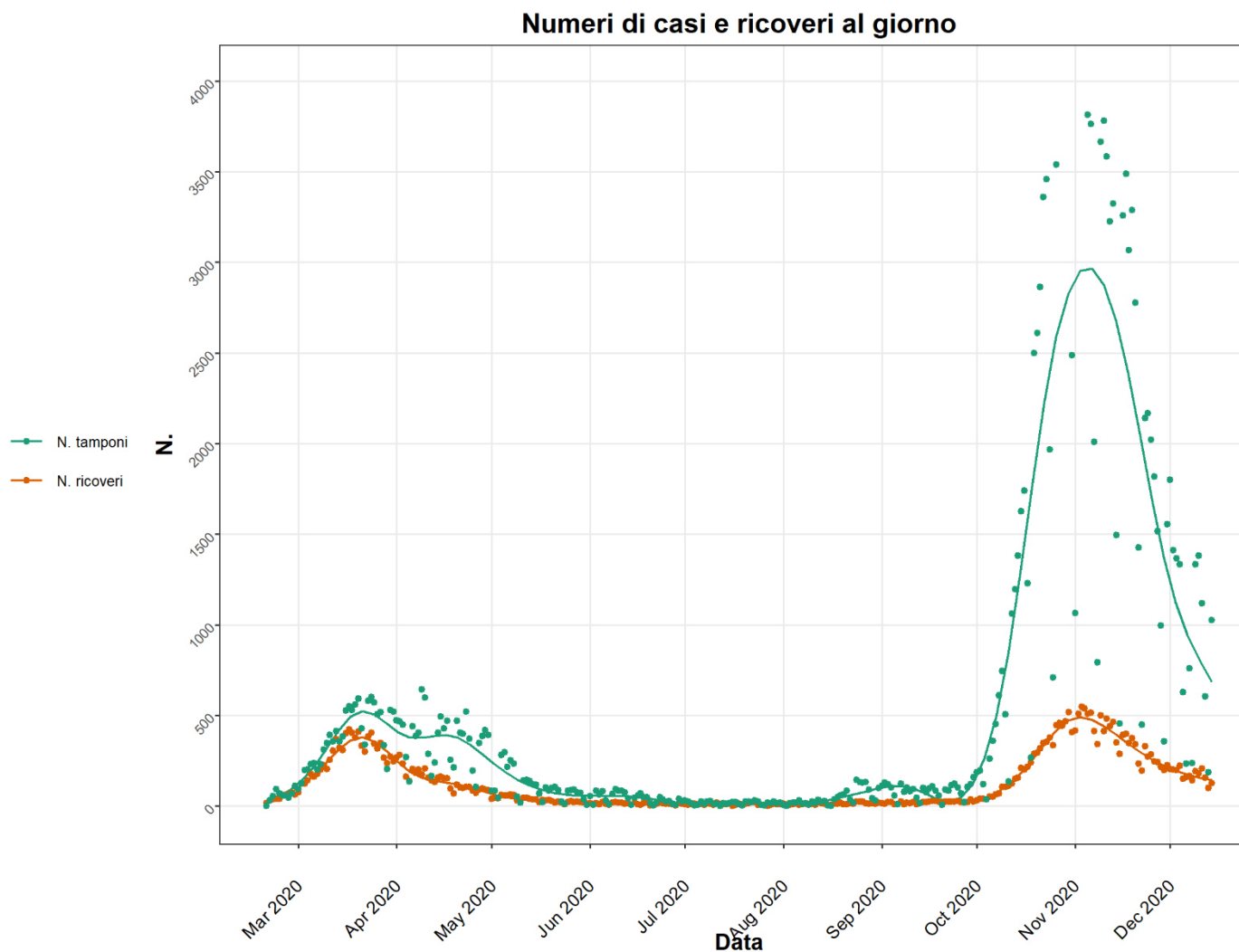
FIG. 1.C NUMERO CASI E RICOVERI GIORNO
