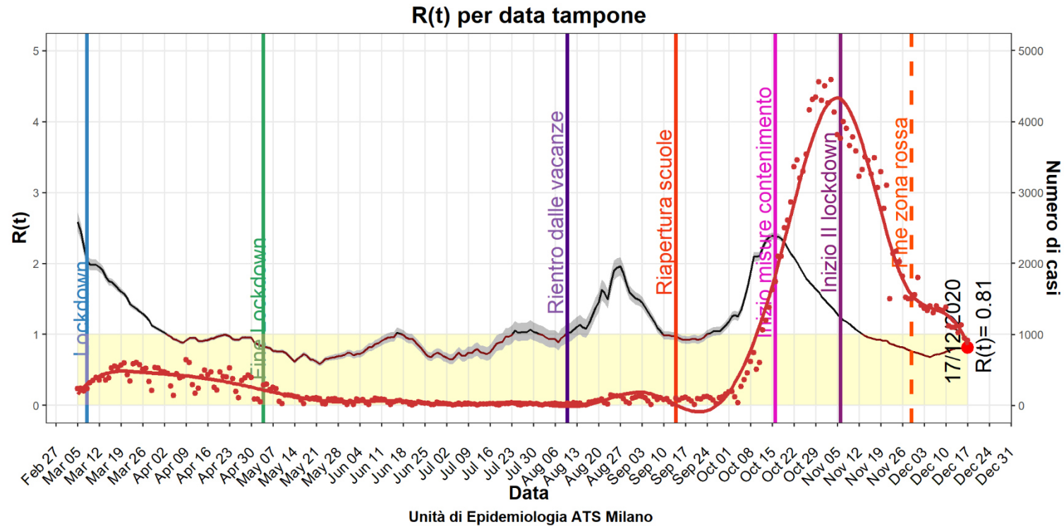
FIG. 1.A R(T) GIORNALIERO PER DATA DI TAMPONE
