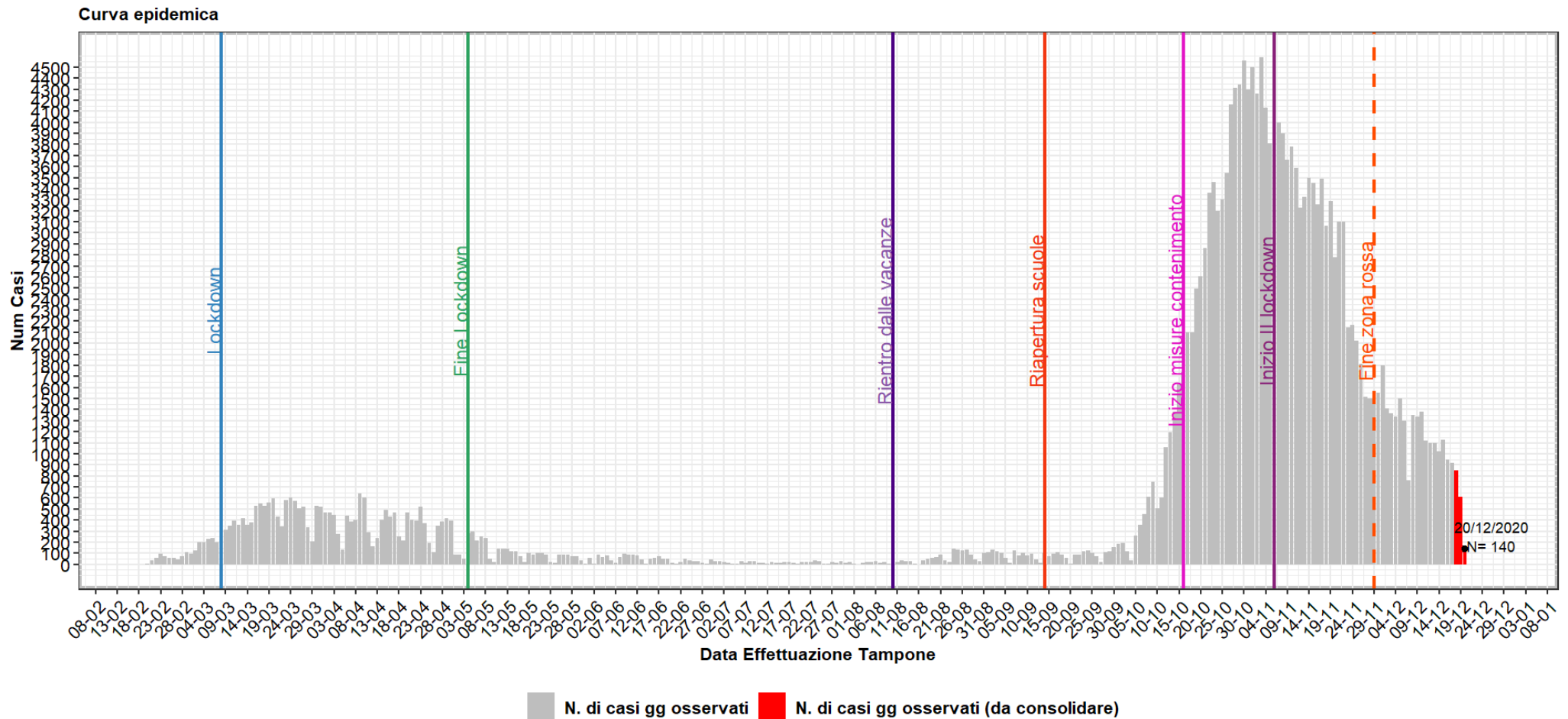
FIG. 6. CURVA EPIDEMICA PER DATA TAMPONE
