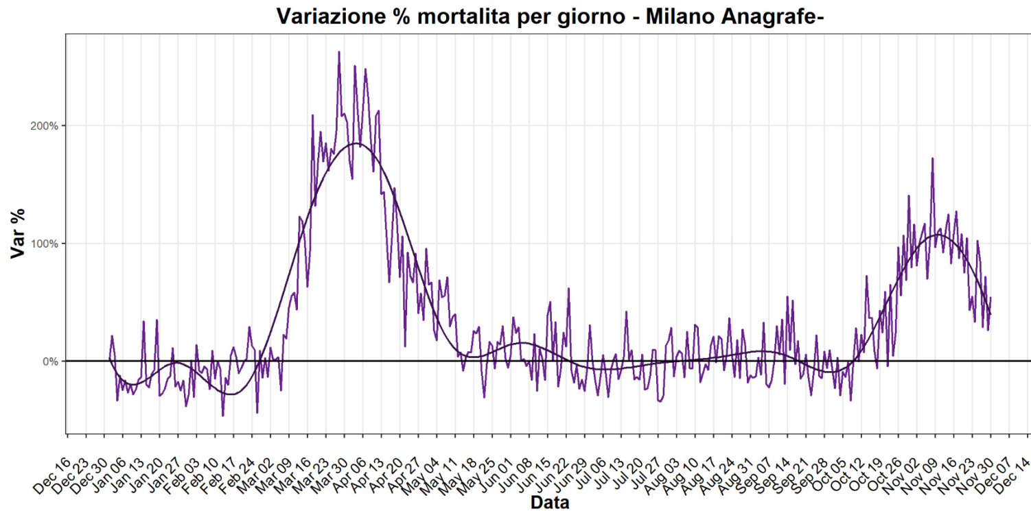
FIG. 1.E VARIAZIONE DELLA MORTALITA' GIORNALIERA SOLO COMUNE DI MILANO
