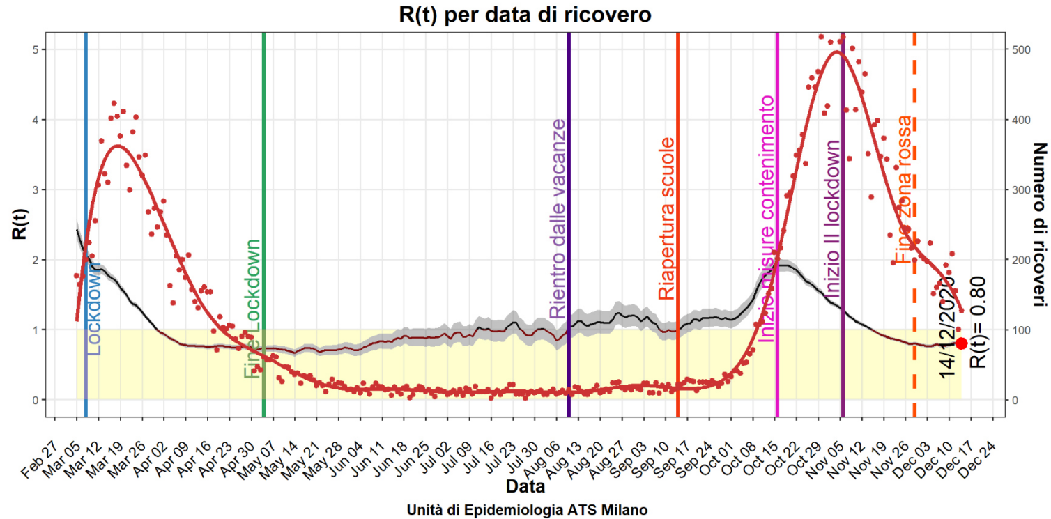
FIG. 1.B R(T) GIORNALIERO PER DATA DI RICOVERO
